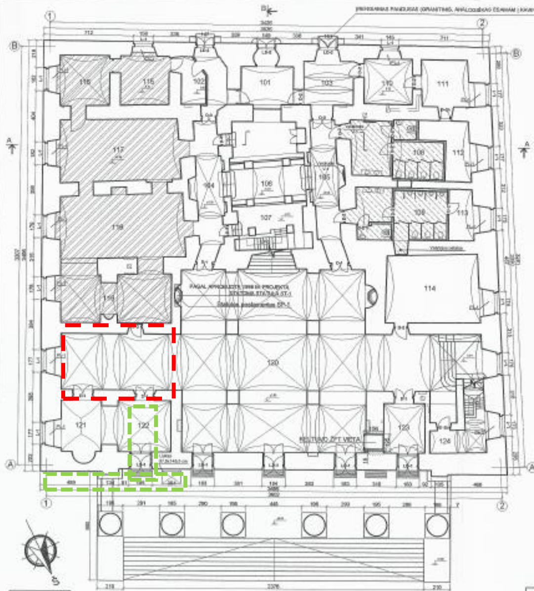
PIRMO AUKŠTO PLANAS M 1:200
